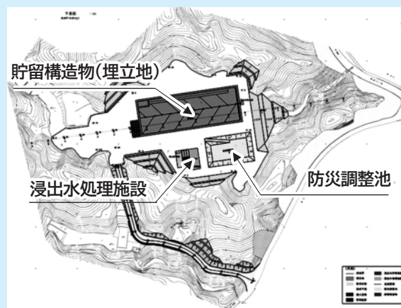
次期広域最終処分場施設配置設計
